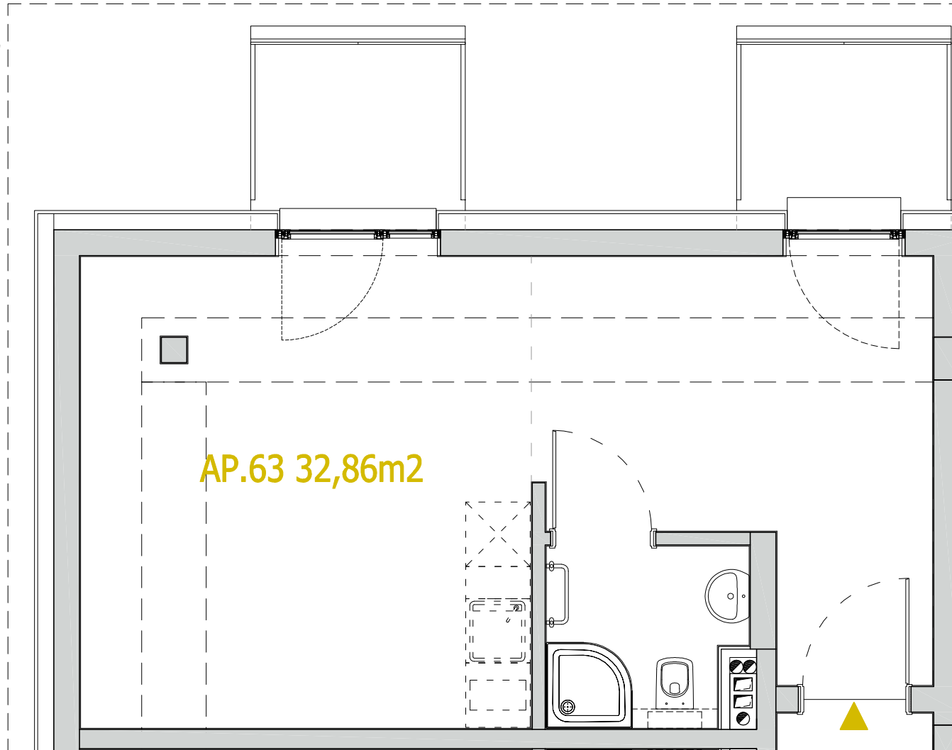
SCHEMAT PIĘTRA
