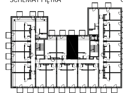
SCHEMAT PIĘTRA
