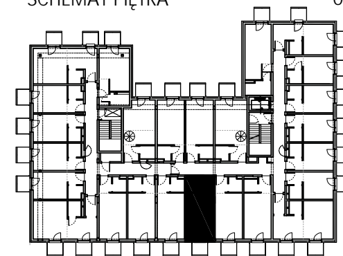
SCHEMAT PIĘTRA 02
