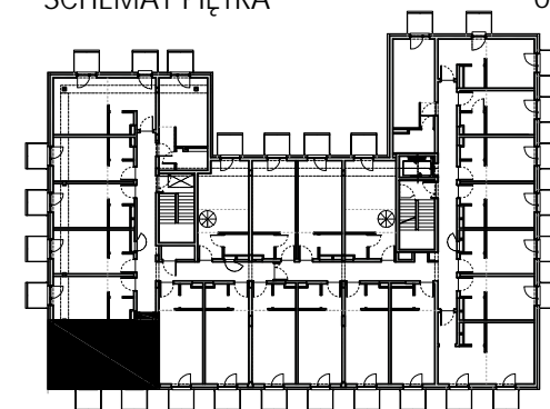
SCHEMAT PIĘTRA
