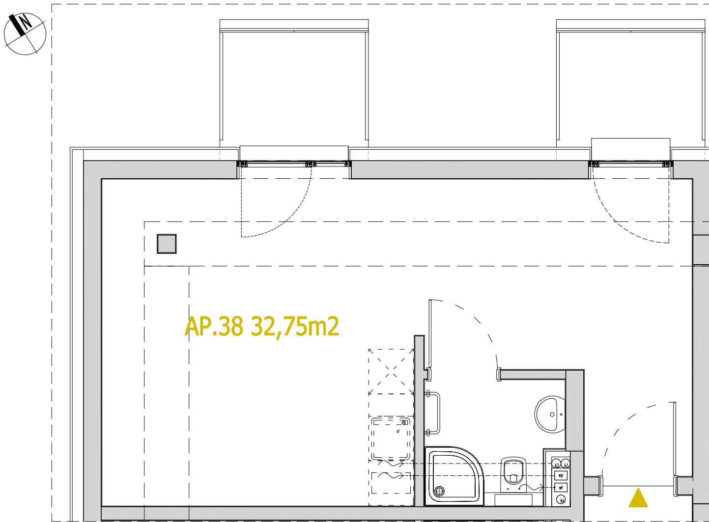
SCHEMAT PIĘTRA
